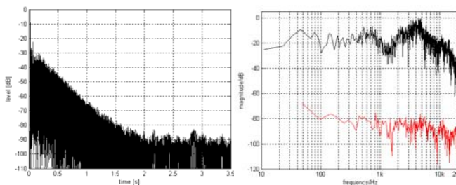
Abbildung 2: am linken Ohr gemessene BRIR, Kopf frontal ausgerichtet (links: ETC, rechts: Raumübertragungsfunktion und Grundstörpektrum)
