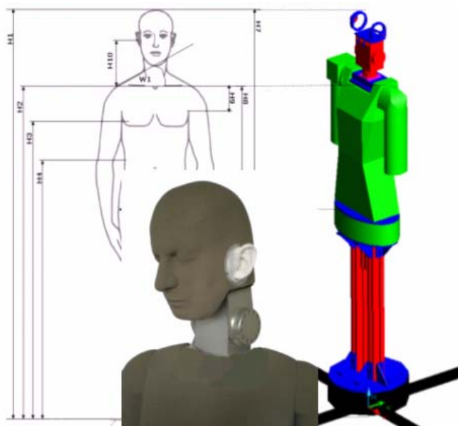
Abbildung 1: Bemaßte anthropometrische Entwurfsvorlage und CAD-Entwurf des modularen Torsos (Farben kennzeichnen unterschiedliche Materialien/Baugruppen)
